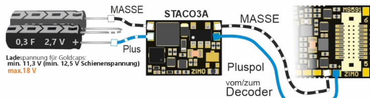
2 Mini-Goldcaps in Serie, STAC03A und Next-Decoder (im Bsp. MS591N18)
