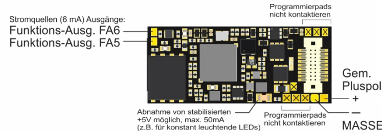
MS580N18 Oberseite, mit Next18 . SOUND
