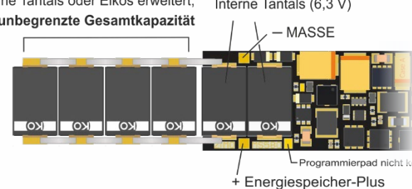
MS580N18 Unterseite, mit opt. externer Erweiterung des Energiespeichers
