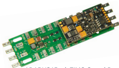
ADAPUS15 mit ZIMO Sound-Decoder MX645P22, 71 x 18 x 7,8 mm
