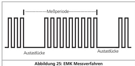
Abbildung 25: EMK Messverfahren
