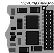
MX640D Oberseite (= wo sich der 21-polige Stecker befindet !)
