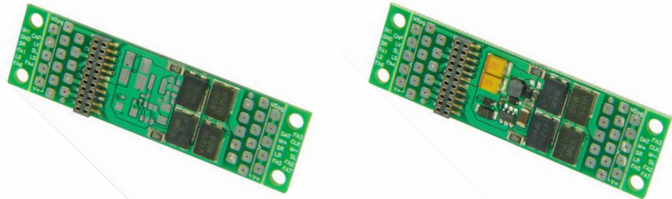
ADAPLU - ohne Niederspannungsquelle ADAPLU15 oder ADAPLU50 - Niederspannung 1,5 bzw. 5V
