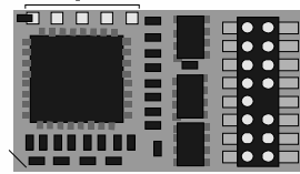
MX630P (mit PluX16)
