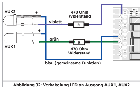
Abbildung 32: Verkabelung LED an Ausgang AUX1, AUX2
