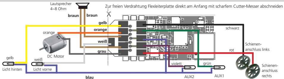
Abbildung 16: Allgemeines Anschlussschema LokSound 5 micro (Beispielverdrahtung, freie Verdrahtung)
