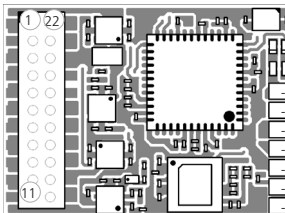
Abbildung 13: LokSound 5 Fx mit 21MTC Schnittstelle
