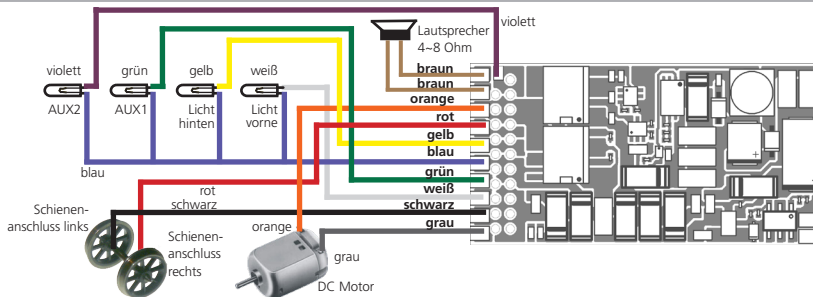
Abbildung 15: Allgemeines Anschlussschema LokSound 5 (Beispielverdrahtung)
