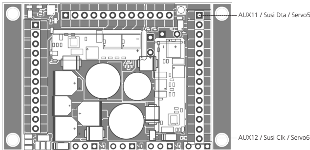
Abbildung 22: LokSound 5 XL Decoder mit Stiftleisten - SUSI Pins für Märklin Lokomotiven
