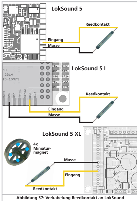
Abbildung 37: Verkabelung Reedkontakt an LokSound
