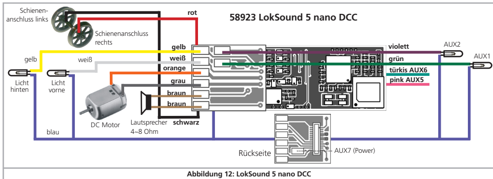
Abbildung 12: LokSound 5 nano DCC
