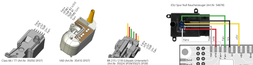
Abbildung 35: Getaktete Raucherzeugermechanik an LokSound 5 L
