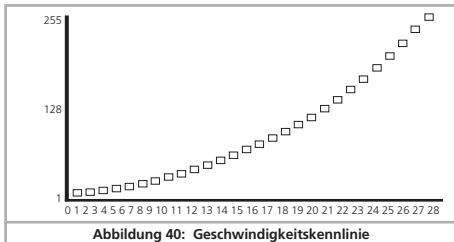
Abbildung 40: Geschwindigkeitskennlinie
