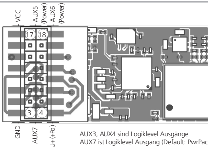
Abbildung 5: LokSound 5 micro PluX16
