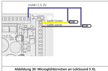
Abbildung 30: Microglühlampen an LokSound 5 XL
