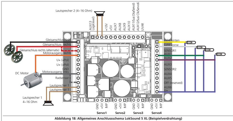
Abbildung 18: Allgemeines Anschlussschema LokSound 5 XL (Beispielverdrahtung)
