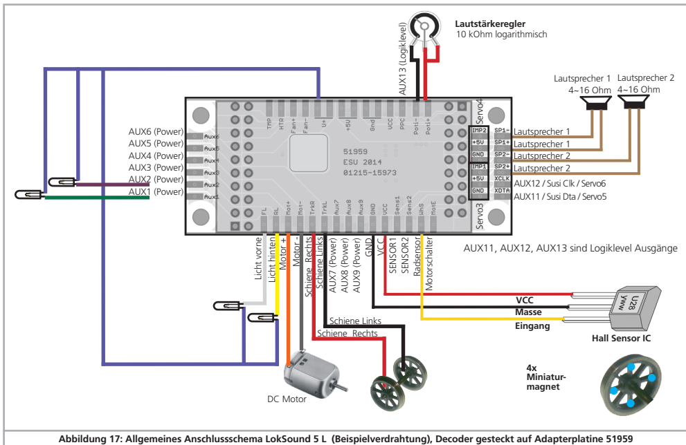
Abbildung 17: Allgemeines Anschlussschema LokSound 5 L (Beispielverdrahtung), Decoder gesteckt auf Adapterplatine 51959
