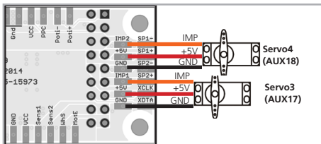
Abbildung 33: RC-Servos an LokSound 5 L
