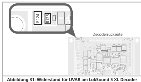
Abbildung 31: Widerstand für UVAR am LokSound 5 XL Decoder
