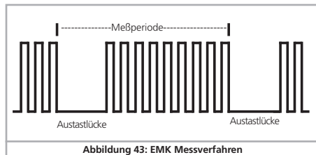
Abbildung 43: EMK Messverfahren
