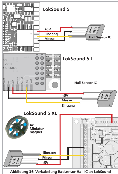
Abbildung 36: Verkabelung Radsensor Hall IC an LokSound
