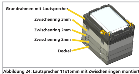
Abbildung 24: Lautsprecher 11x15mm mit Zwischenringen montiert
