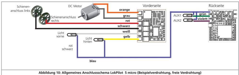
Abbildung 10: Allgemeines Anschlussschema LokPilot 5 micro (Beispielverdrahtung, freie Verdrahtung)
