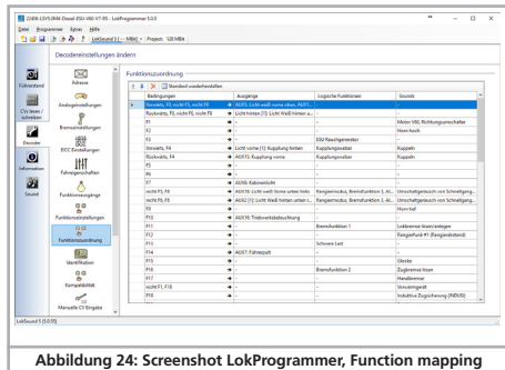
Abbildung 24: Screenshot LokProgrammer, Function mapping
