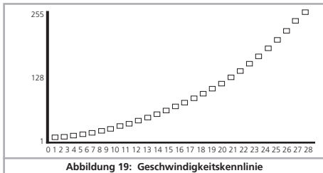
Abbildung 19: Geschwindigkeitskennlinie
