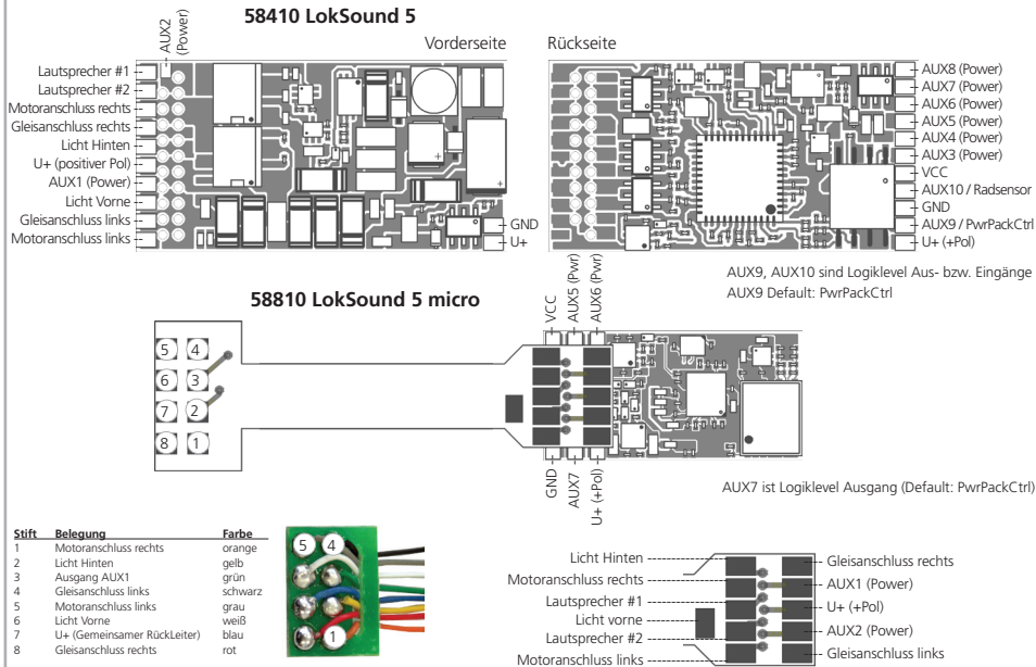
Abbildung 1: LokSound 5 & LokSound 5 micro mit 8-poliger NEM652 Schnittstelle
