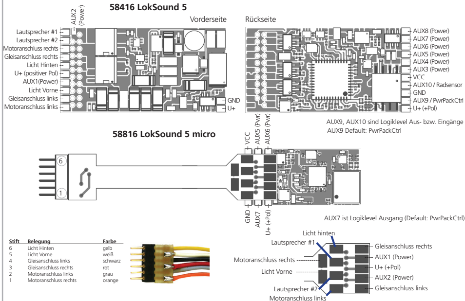
Abbildung 2: LokSound 5 & LokSound 5 micro mit 6-poliger NEM651 Schnittstelle
