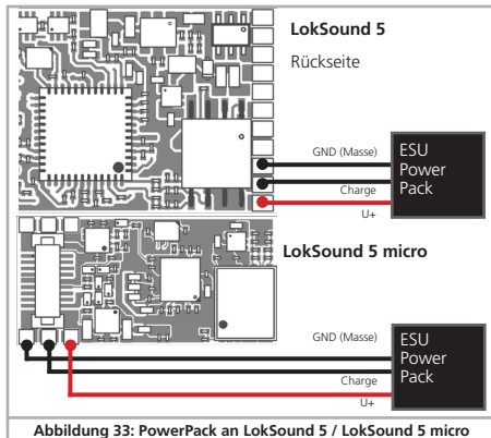
Abbildung 33: PowerPack an LokSound 5 / LokSound 5 micro
