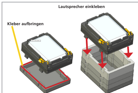
Abbildung 20: Lautsprecher 11x15mm mit Zwischenringen montiert
