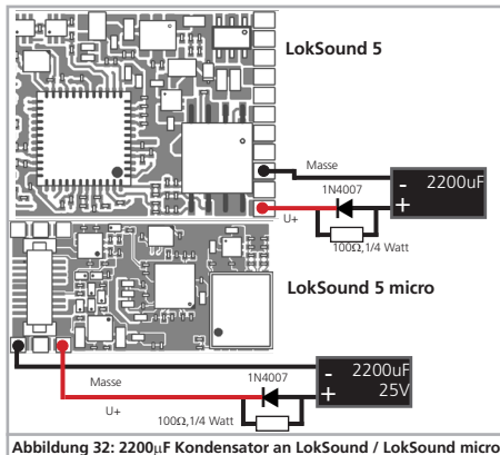
Abbildung 32: 2200µF Kondensator an LokSound / LokSound micro
