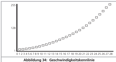
Abbildung 34: Geschwindigkeitskennlinie
