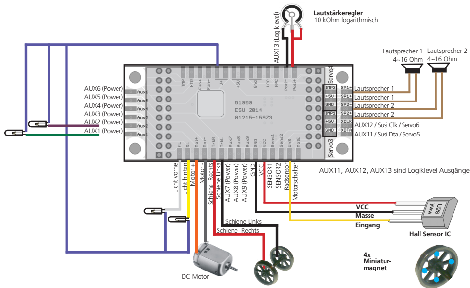
Abbildung 11: Allgemeines Anschlussschema LokSound 5 L (Beispielverdrahtung), Decoder gesteckt auf Adapterplatine 51959
