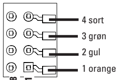
Loddepads oppe
