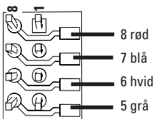
Loddepads nede
