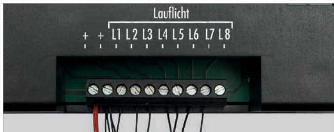
Abb. 22: Warnlichter/Baustellensicherung anschließen
