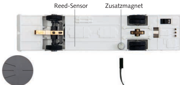
Abb. 26: Unterboden H0
